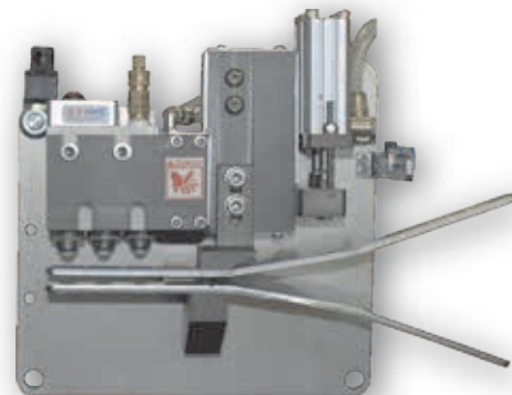
Beleimungsstation mit kontaktlosem Dreifach-Ventil
