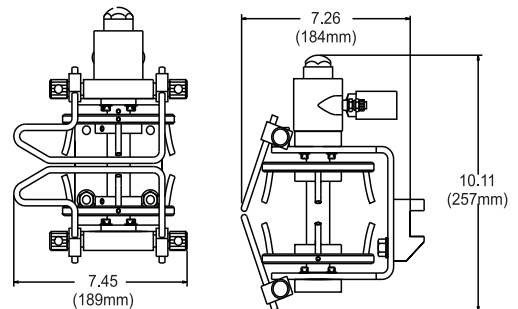
582x586 TR500M Pneumatisches Stanzreste-Entfernersystem, maximal 30 psi
