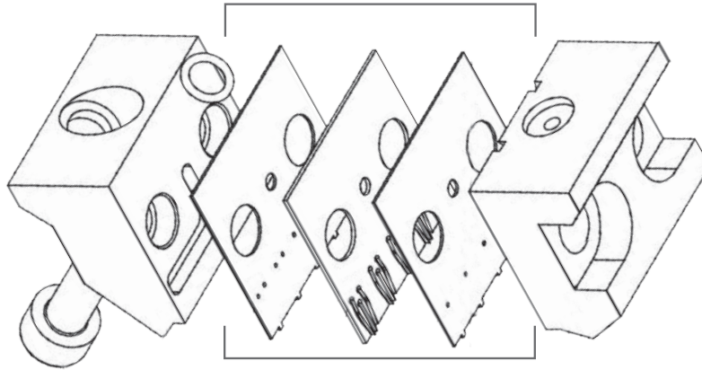
Konstruktion auf Basis von Zwischenscheiben aus Edelstahl
