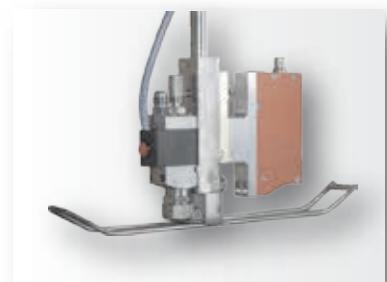
Kontaktlose Version mit Leimmuster-Kontrolle
