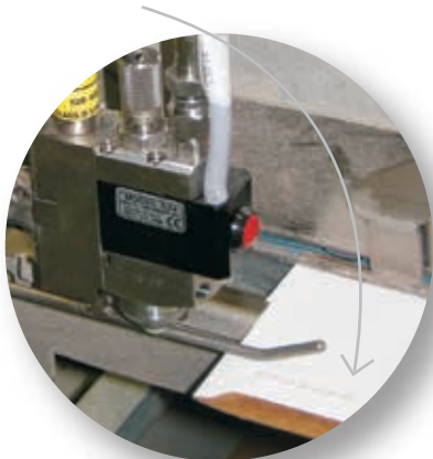
Ventil 524 beim Auftragen von Leimpunkten in einer Faltkarton-Klebmaschine
